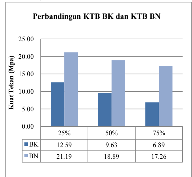
Gambar.5.Histogram perbandingan hasil uji kuat tekan beton biji karet dengan beton korat ayak 25%, 50% dan 75% pada umur pengujian 28 hari
