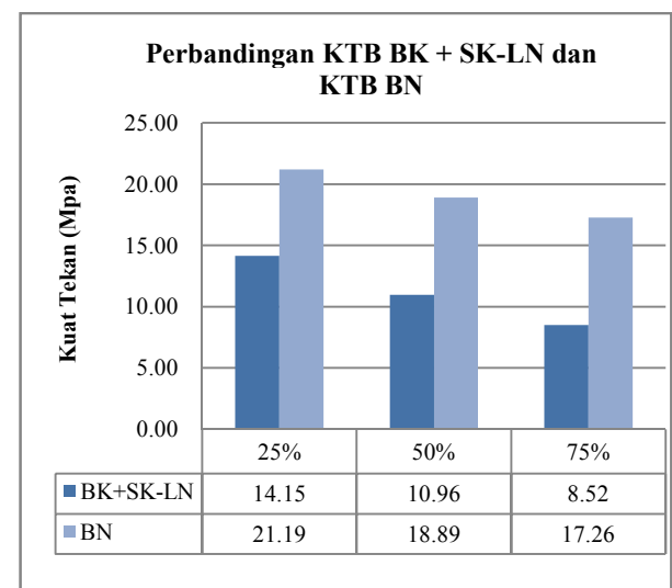
Gambar.6.Histogram perbandingan hasil uji kuat tekan beton biji karet+Sikament-LN dengan beton korat ayak 25%, 50% dan 75% pada umur pengujian 28 hari
