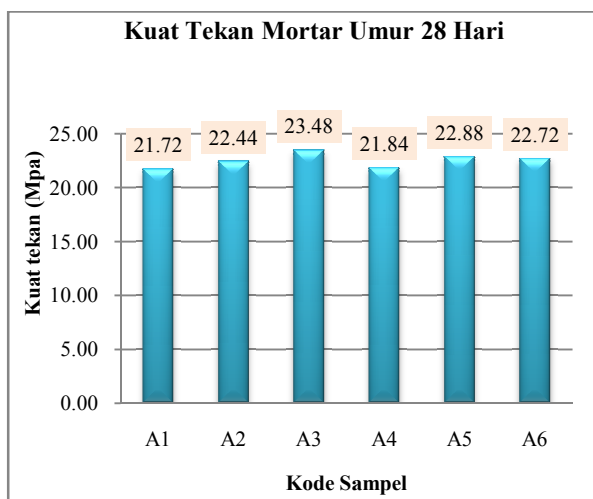
Gambar.4.Histogram hasil uji kuat tekan mortar pada umur pengujian 28 hari
