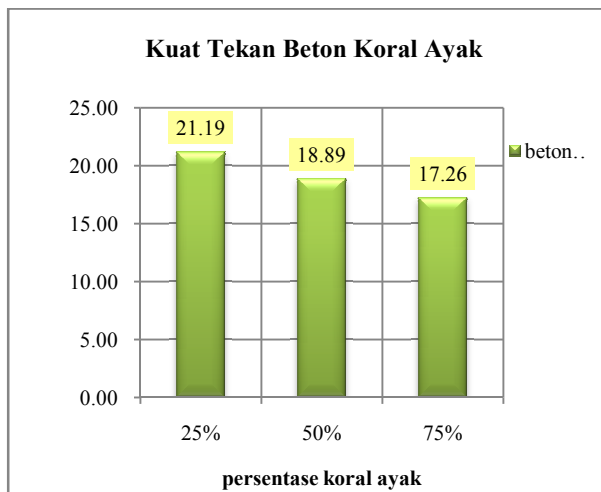
Gambar.3.Histogram hasil uji kuat tekan beton korat ayak 25%, 50% dan 75% pada umur pengujian 28 hari
