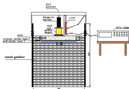
Gambar 1. Pemodelan Benda Uji
