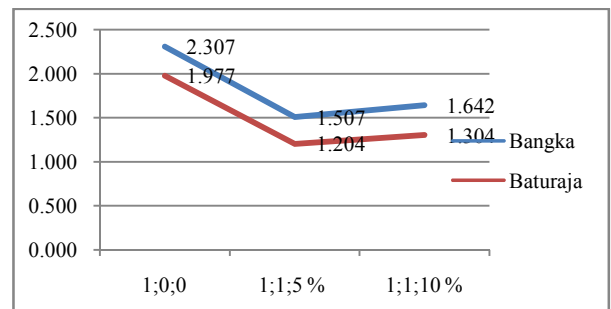
Grafik perubahan berat jenis umur 7 hari
