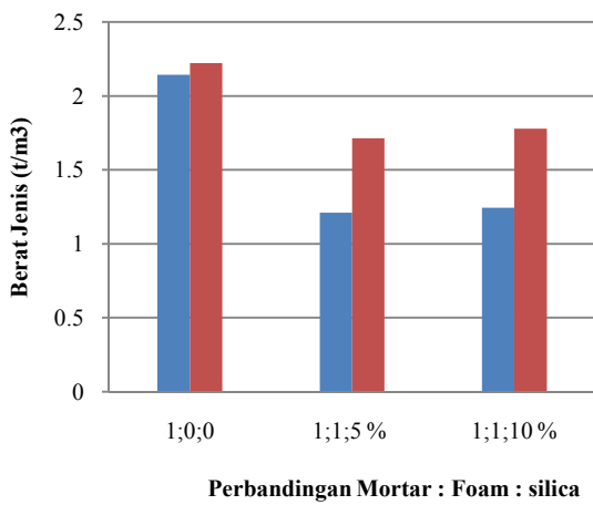
Grafik perubahan berat jenis pada umur 3 hari
