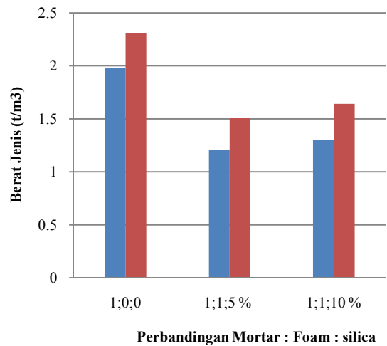
Grafik perubahan berat jenis umur 7 hari
