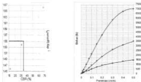
Gambar 3.10. CBR Desain dan Hasil Dari Pengujian CBR
