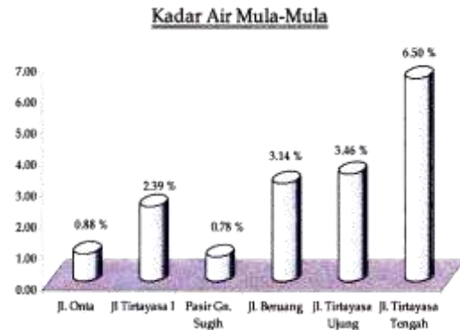
Gambar 3.1 Kadar air mula
