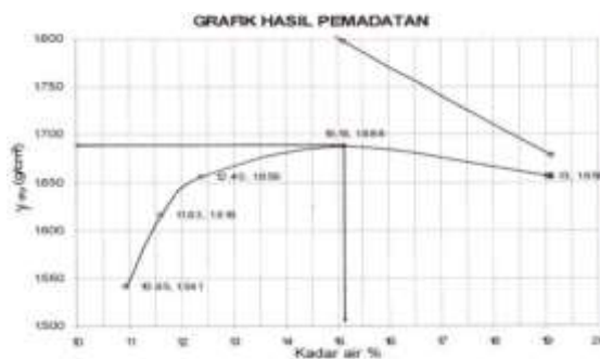
Gambar 3.8. Hasil Pemadatan Jl. Onta
