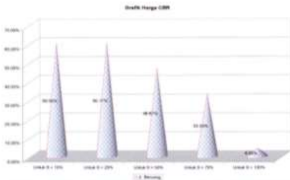
Gambar 3.15 Nilai CBR Terhadap Derajat Kejenuhan Jl. Beruang
