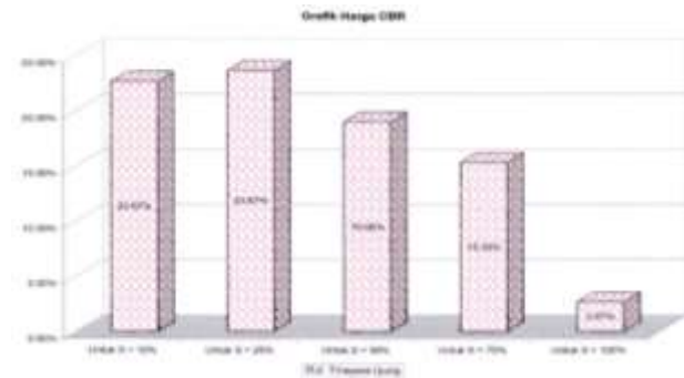
Gambar 3.14. Nilai CBR Terhadap Derajat Kejuhanan Jl. Tirtayasa Ujung
