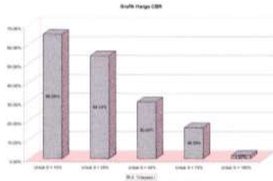
Gambar 3.13. Nilai CBR Terhadap Derajat Kejuhanan Pasir Gn Sugih
