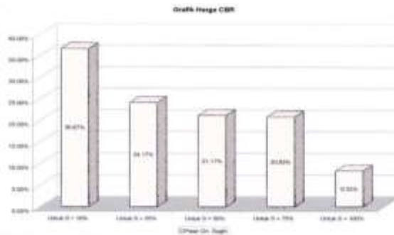
Gambar 3.12. Nilai CBR Terhadap Derajat Kejuhanan Jl. Tirtayasa I
