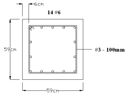
Gambar 16. Penulangan Kolom
