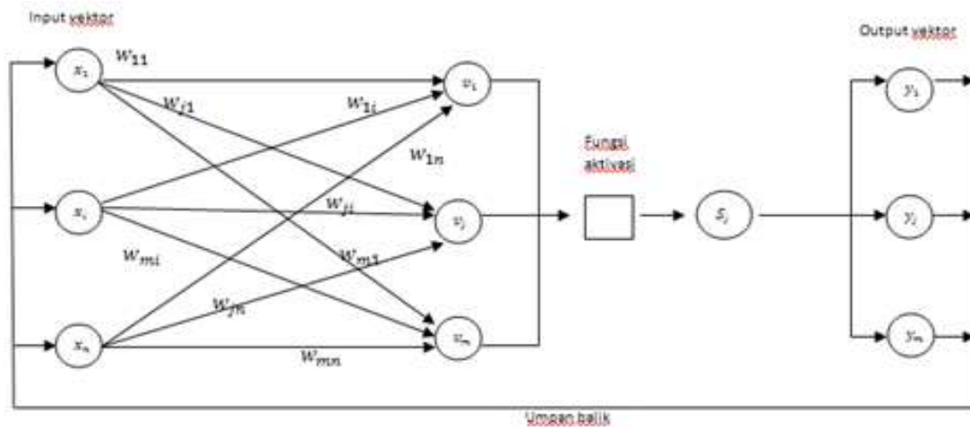
Gambar 1. Arsitektur Jaringan Hopfield
