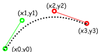
Gambar 1. Titik-titik pada kurva Bezier[18]
