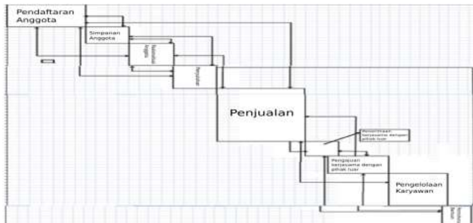
Gambar 4. Arsitektur Informasi
