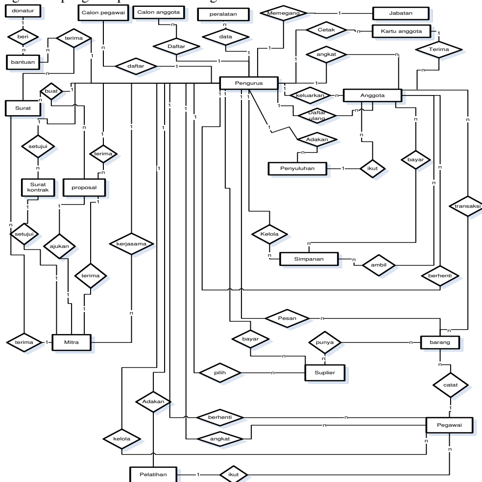
Gambar 5. ER Diagram
