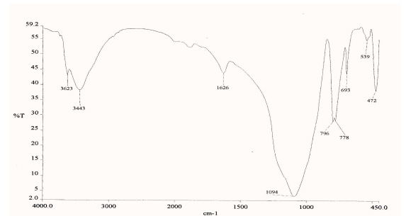
Gambar 3 Spektra inframerah lempung B
