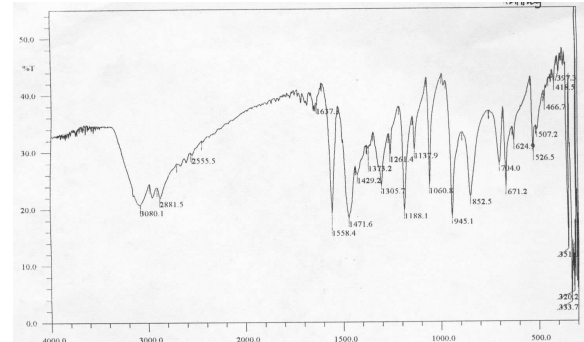
Gambar 4. Spektra inframerah 3-merkpto-1,2,4triazol (TRZSH)
