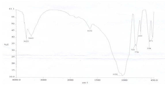
Gambar 2 Spektra inframerah lempung A
