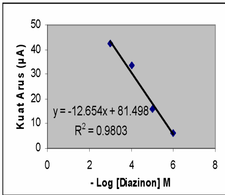
Gambar 2. Plot [Diazinon] vs Kuat Arus Komposisi membran 10/10 %.
