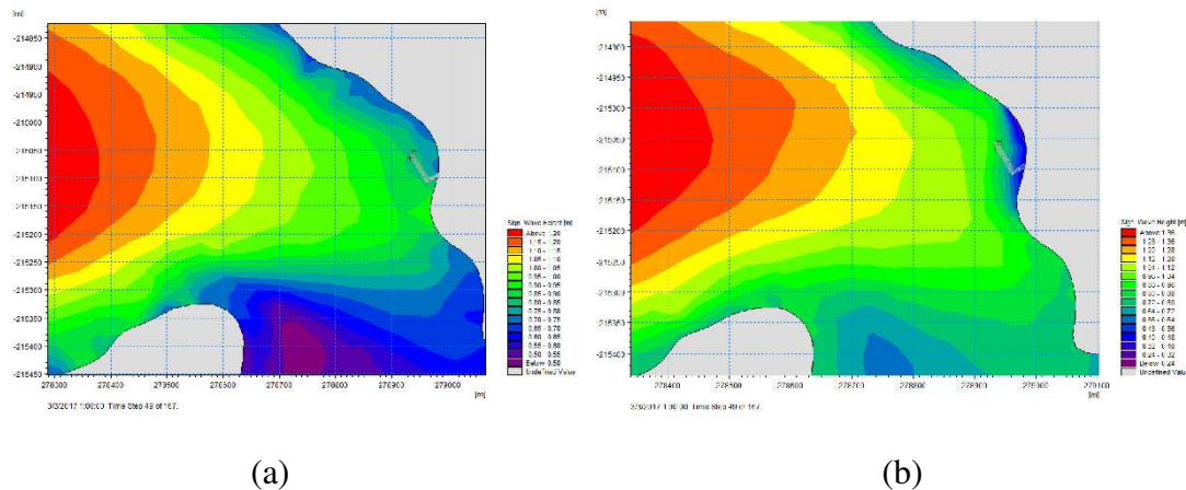
Gambar 5 Hasil Pemodelan Gelombang (a) H_{1\%} , (b) H_{max} Kala Ulang
