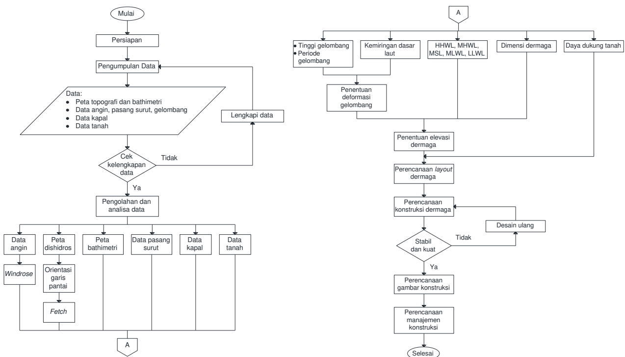
Gambar 2 Flowchart Perencanaan Dermaga Perintis Wakde
