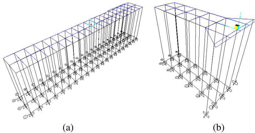
Gambar 11 Pemodelan Struktur (a) Dermaga dan (b) Trestle pada Program SAP 2000
