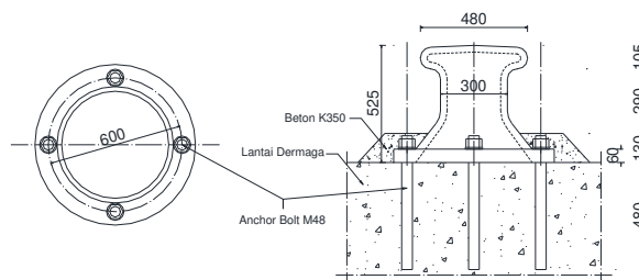
Gambar 10 Bitt Kapasitas 25 ton
