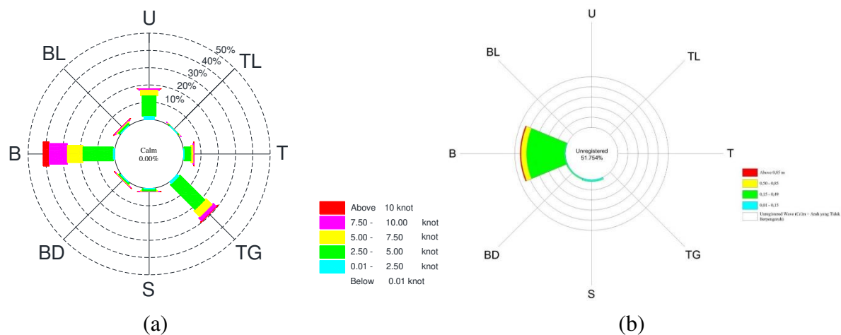
Gambar 3 (a) Windrose dan (b) Waverose Dermaga Perintis Wakde Tahun 2001 -2006
