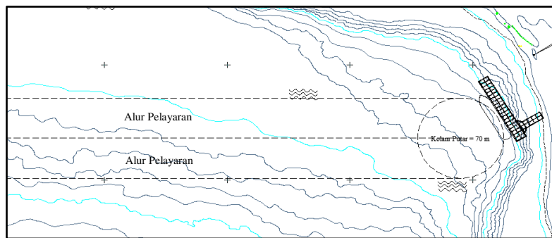
Gambar 8 Hasil Perencanaan Layout Pelabuhan
