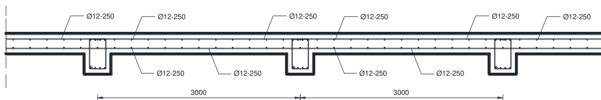
Gambar 12 Penulangan Memanjang pada Pelat Lantai Dermaga
