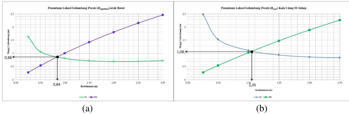
Gambar 4 Grafik Penentuan Lokasi Gelombang Pecah dengan (a) H_{1\%} , (b) H Kala Ulang
