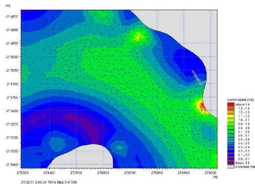
Gambar 7 Pemodelan Arus di Lokasi Dermaga
