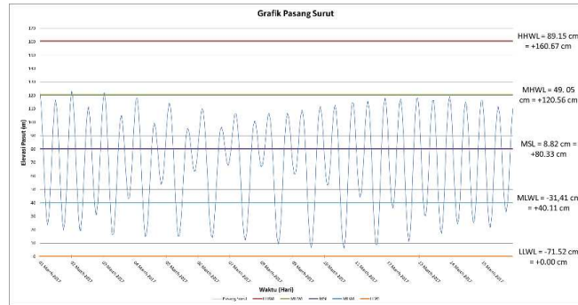
Gambar 6 Grafik Pasang Surut dengan Metode Admiralty
