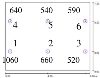
Gambar 9: Tingkat intensitas cahaya pada gedung Marwah lantai 3 Sore
