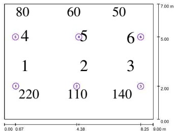
Gambar 13: Tingkat intensitas cahaya pada gedun Madinah lantai 1 pagi hari
