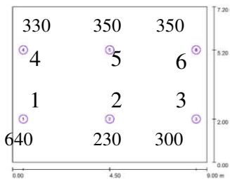
Gambar 12: Tingkat intensitas cahaya pada gedung Marwah lantai 4 Sore
