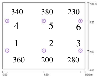
Gambar 4: Tingkat intensitas cahaya pada gedung Marwah lantai 2 pagi
