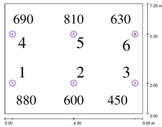
Gambar 8: Tingkat intensitas cahaya pada gedung Marwah lantai 3 siang
