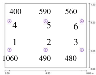
Gambar 6: Tingkat intensitas cahaya pada gedung Marwah lantai 2 Sore
