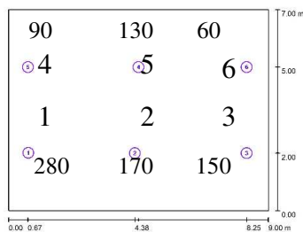
Gambar 16: Tingkat intensitas cahaya pada gedun Madinah lantai 2 pagi
