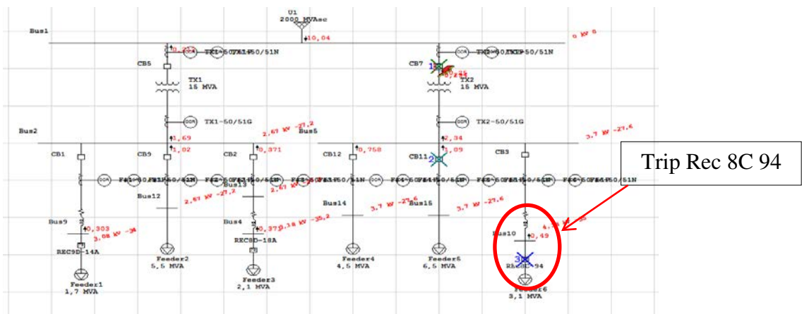
Gambar 4.7 Simulasi ETAP 12.6.0 Gardu Induk 6D Rec 8C 94 Trip
