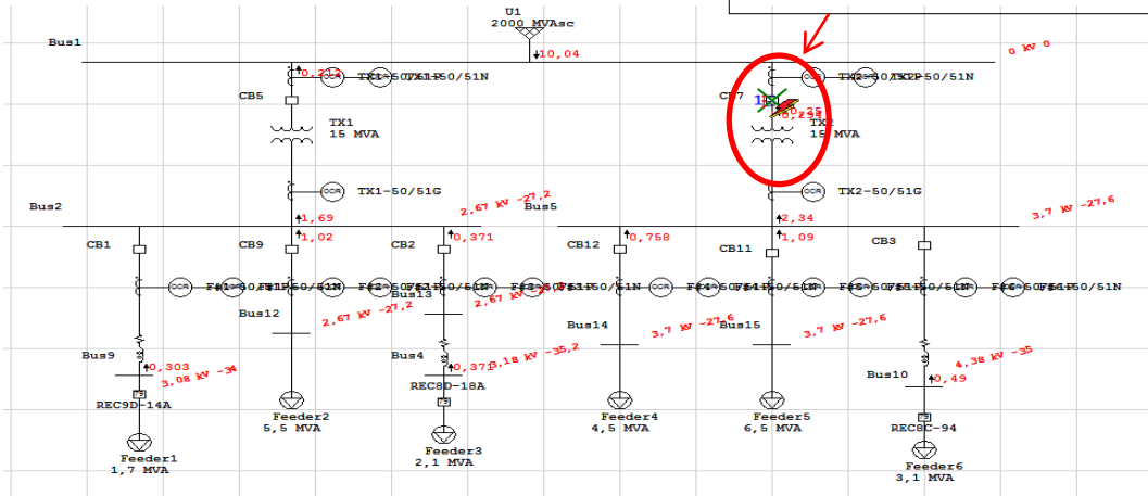
Gambar 4.5 Simulasi ETAP 12.6.0 Gardu Induk 6D CB7 Trip
