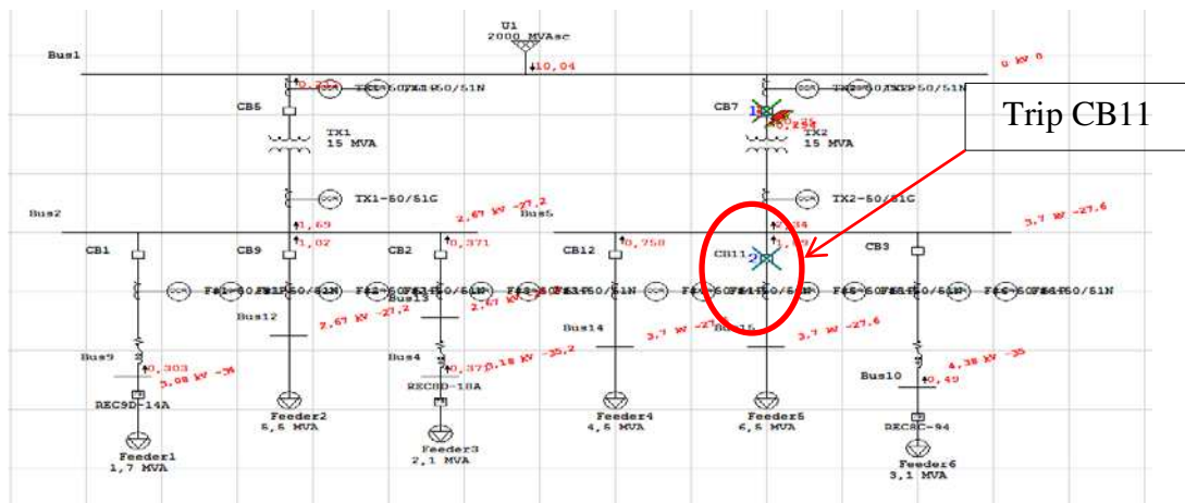
Gambar 4.6 Simulasi ETAP 12.6.0 Gardu Induk 6D CB11 Trip
