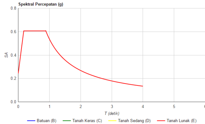
Gambar 1. Grafik Respon Spektrum Temanggung (Tanah Lunak)
