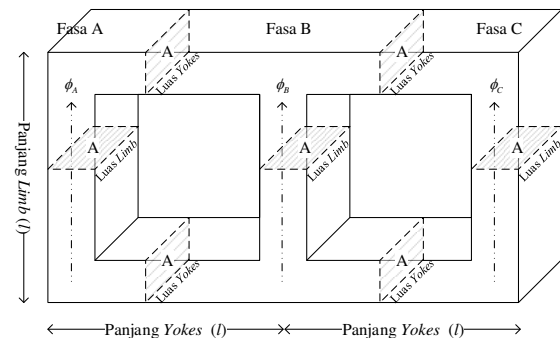
Gambar 4. Konstruksi inti besi transformator tiga fasa tiga lengan
