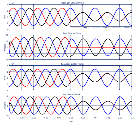
Gambar 17. Karakteristik tegangan dan arus primer saat open-circuit beban 100%
