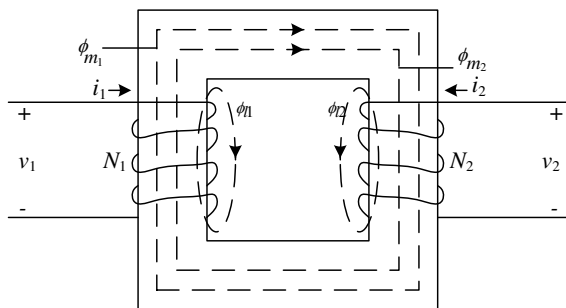
Gambar 2. Rangkaian Magnetik Transformator
