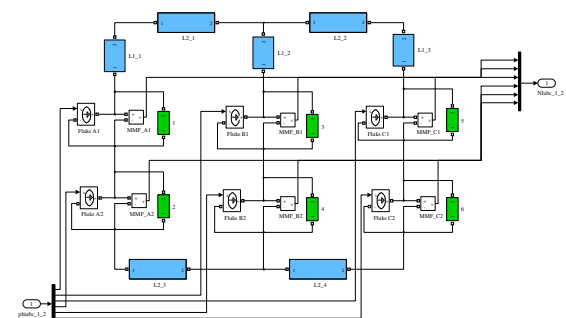
Gambar 10. Model keseluruhan simulink rangkaian magnetik pada inti besi transformator tiga fasa
