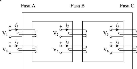
Gambar 3. Konstuksi transformator tiga lengan
