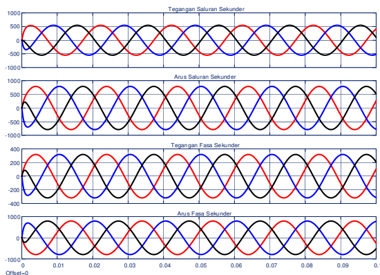
Gambar 15. Karakteristik tegangan dan arus sekunder saat normal beban 100%
