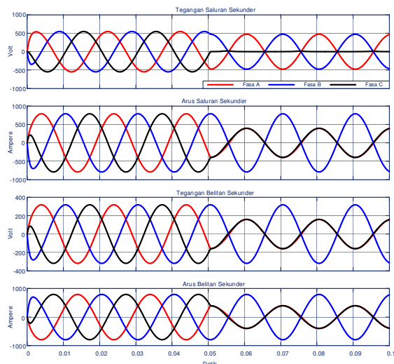
Gambar 18. Karakteristik tegangan dan arus sekunder saat open-circuit beban 100%
