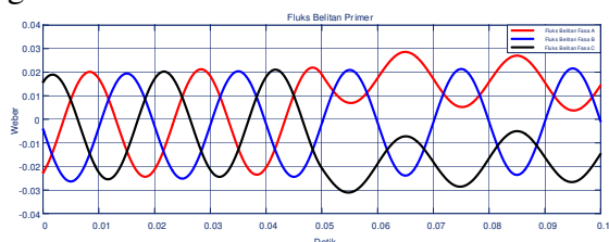
Gambar 19. Karakteristik fluks magnet saat open-circuit beban 100%
