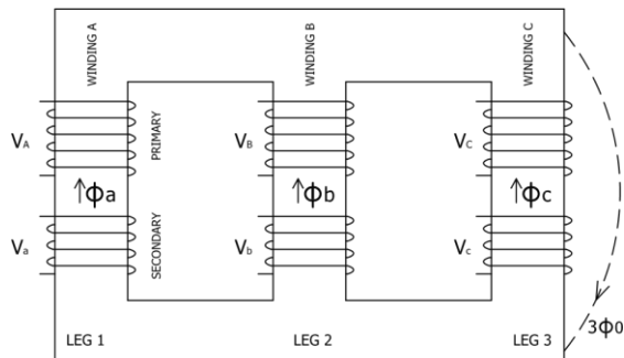
Gambar 1. Konstuksi transformator tiga lengan
