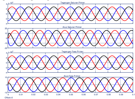
Gambar 14. Karakteristik tegangan dan arus primer saat normal beban 100%
