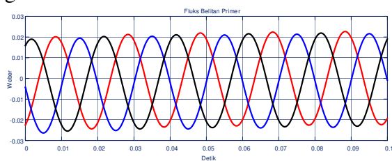
Gambar 16. Karakteristik fluks magnet saat normal beban 100%
