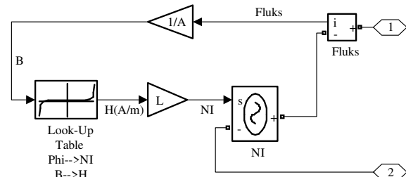
Gambar 8. Model simulink hubungan karakteristik B – H Curve yoke dan core pada inti besi transformator
