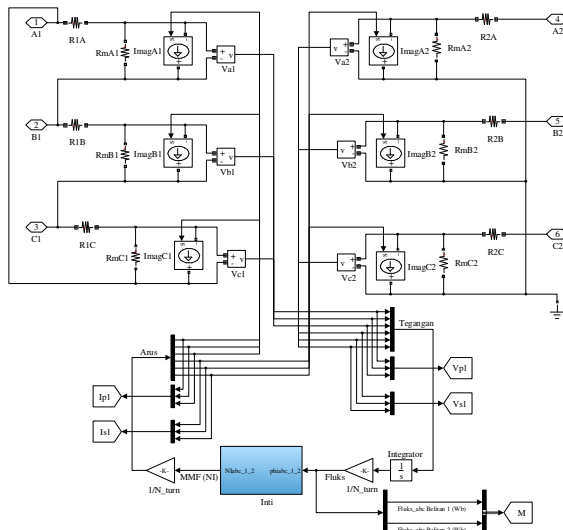
Gambar 12. Rangkaian keseluruhan model transformator tiga fasa tiga lengan
