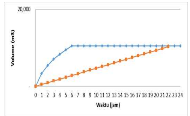
Gambar 8. Hubungan kapasitas tampungan dengan pompa 0,13 m 3 /detik terhadap waktu.
