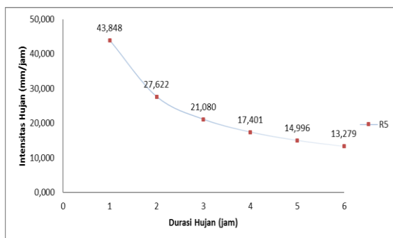
Gambar 4. Kurva Intensitas Curah Hujan.
