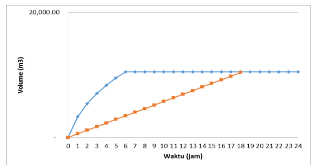
Gambar 9. Hubungan kapasitas tampungan dengan pompa 0,75 m 3 /detik terhadap waktu.
