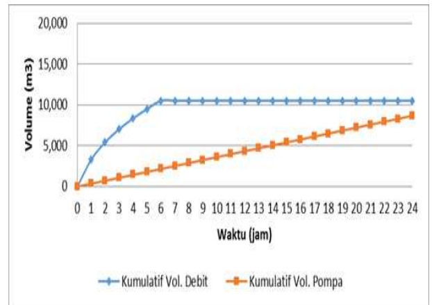
Gambar 7. Hubungan kapasitas tampungan dengan pompa 0,1 m 3 /detik terhadap waktu
