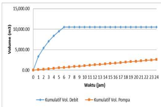
Gambar 6. Hubungan kapasitas tampungan dengan pompa 0,03 m 3 /detik terhadap waktu.
