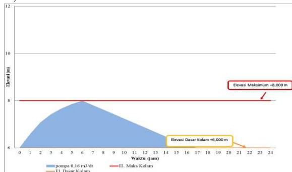
Gambar 10. Simulasi Pompa Kala Ulang 5 tahun dengan kapasitas 0,16 m 3 /detik.
