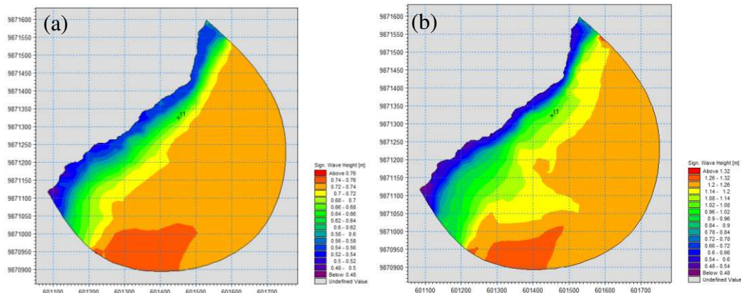
Gambar 5 Hasil Pemodelan Gelombang (a) H_{33\%} , (b) H_{max} Kala Ulang
