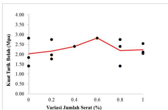
Gambar 8. Hasil pengujian kuat tarik belah beton umur 28 hari.
