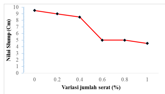
Gambar 6. Hasil Pengujian Slump
