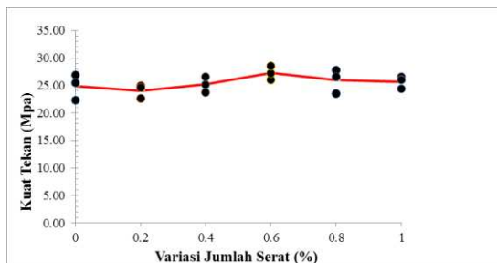
Gambar 7. Hasil pengujian kuat Tekan beton umur 28 hari
