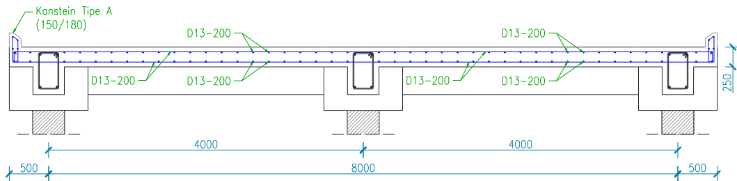
Gambar 11 – Penulangan pada pelat lantai
