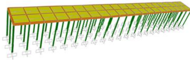
Gambar 10 Pemodelan struktur dermaga pada program SAP 2000
