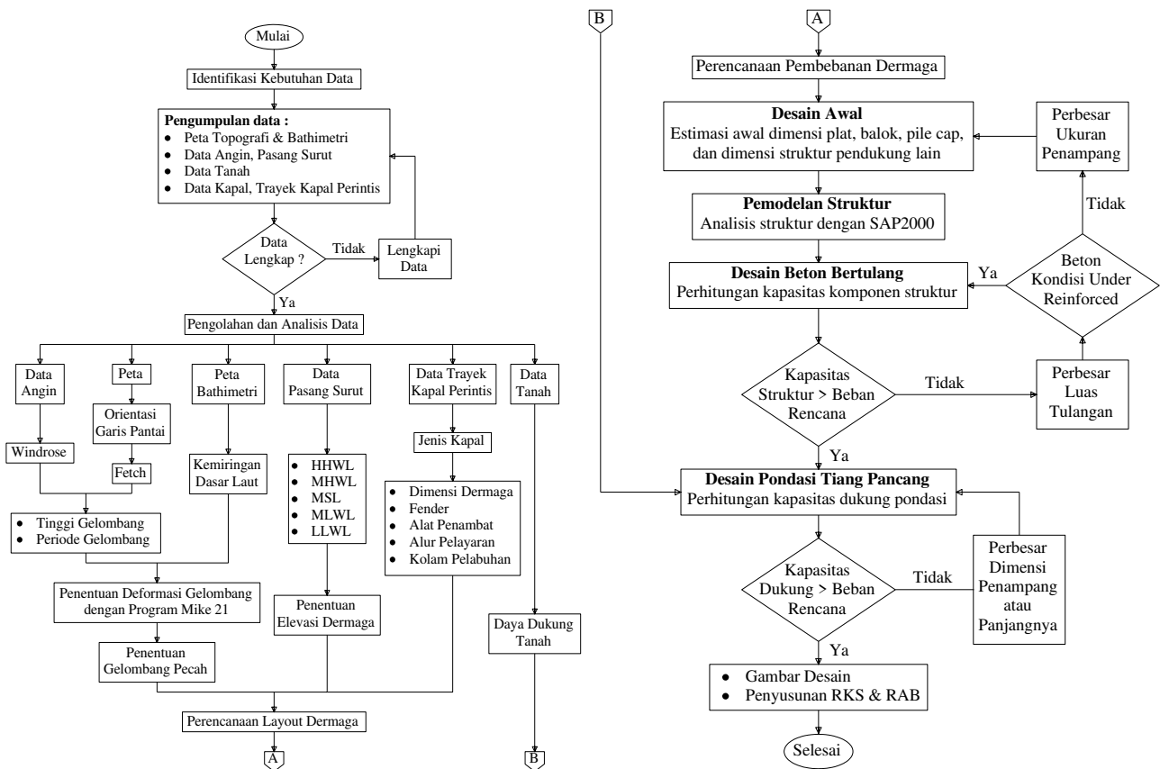
Gambar 2 Flowchart perencanaan dermaga kapal perintis Pulau Kurudu
