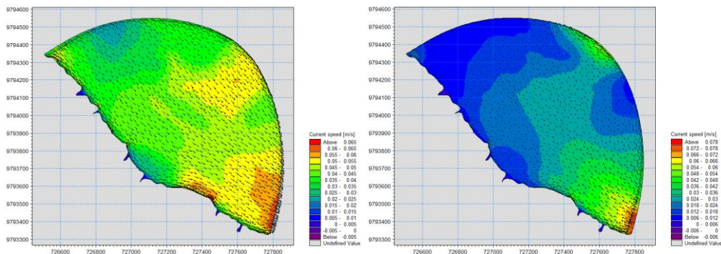
Gambar 7 Distribusi kecepatan arus pasang surut pada kondisi (a) surut menuju pasang, (b) pasang menuju surut
