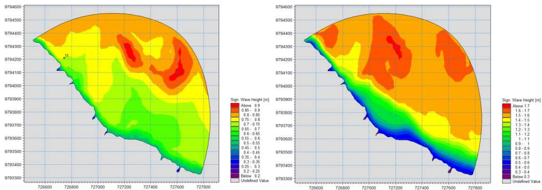
Gambar 5 Hasil pemodelan gelombang (a) H_{33\%} , (b) H_{\max} kala ulang
