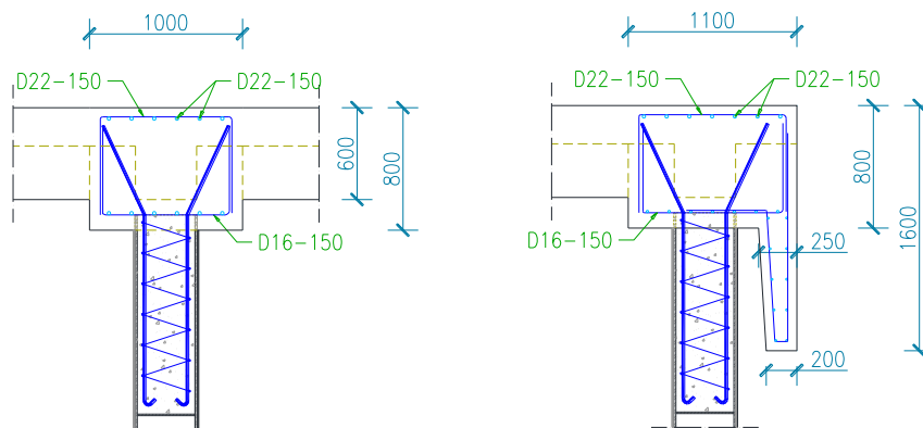
Gambar 12 Penulangan pada pile cap
