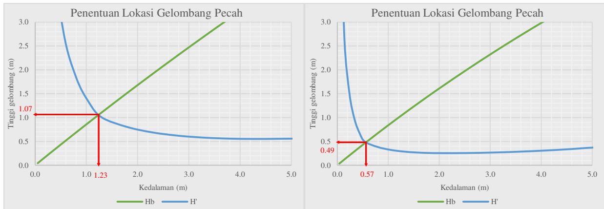
Gambar 4 Grafik penentuan lokasi gelombang pecah dengan (a) H_{\max} kala ulang, (b) H_{33\%}
