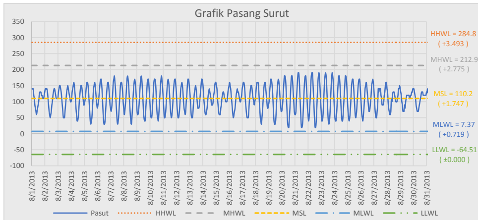
Gambar 6 Grafik pasang surut dengan metode admiralty
