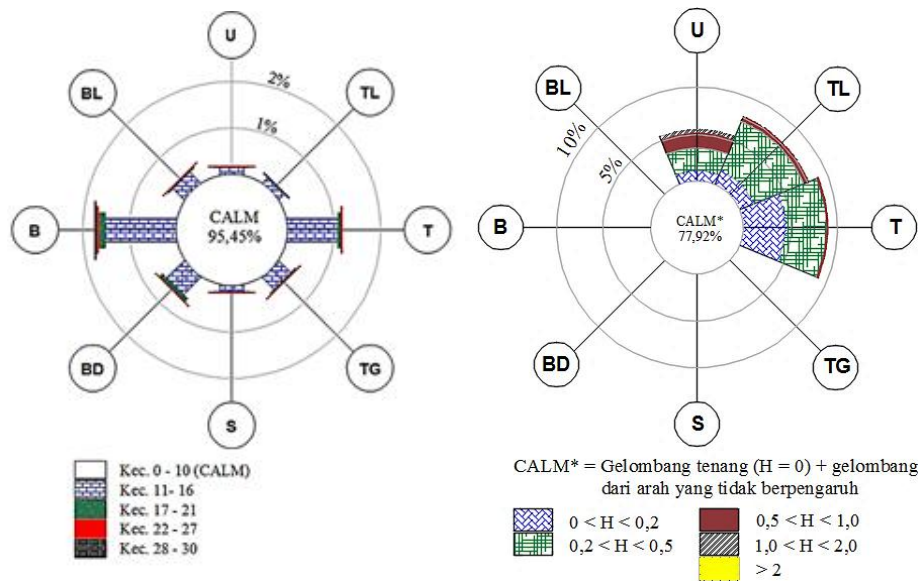
Gambar 3 Windrose dan waverose Tahun 1999 – 2016
