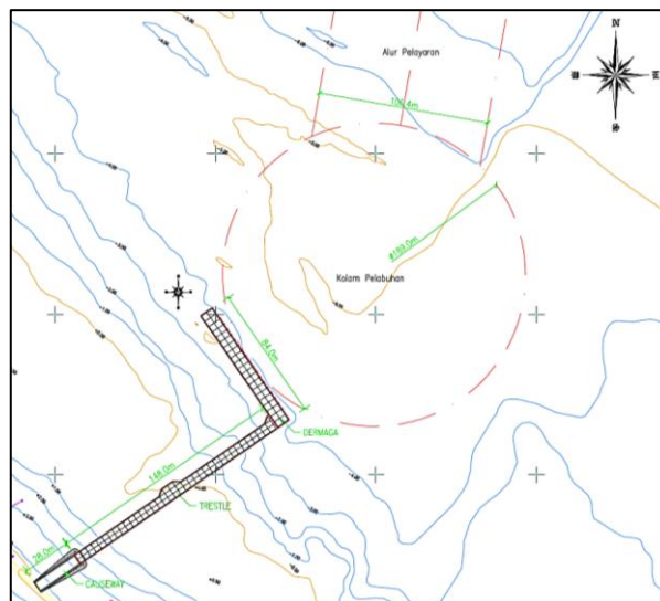
Gambar 8 Hasil perencanaan layout pelabuhan
