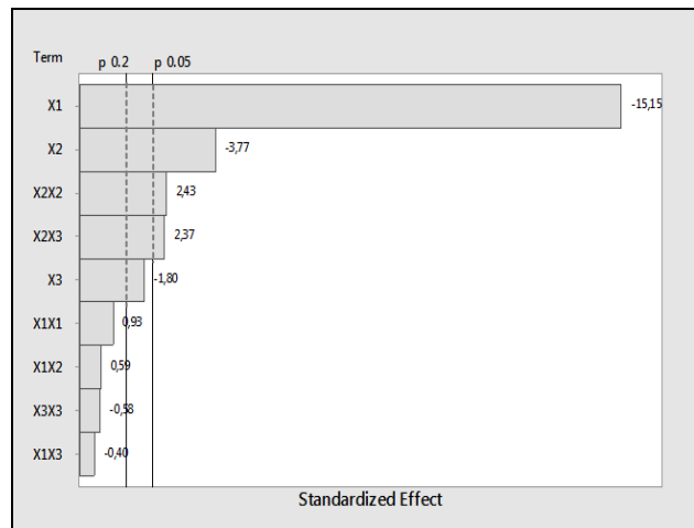
Gambar 3. Diagram Pareto Pengaruh Kondisi Proses terhadap Kadar Lignin Pulp
