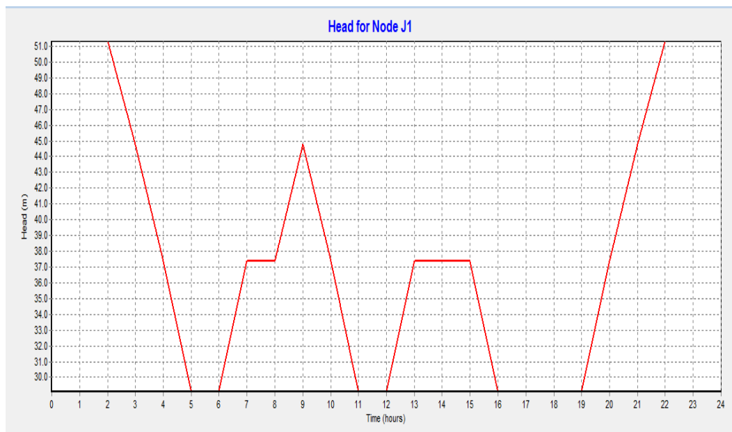
Gambar 7 Grafik Head pada Junction J1
