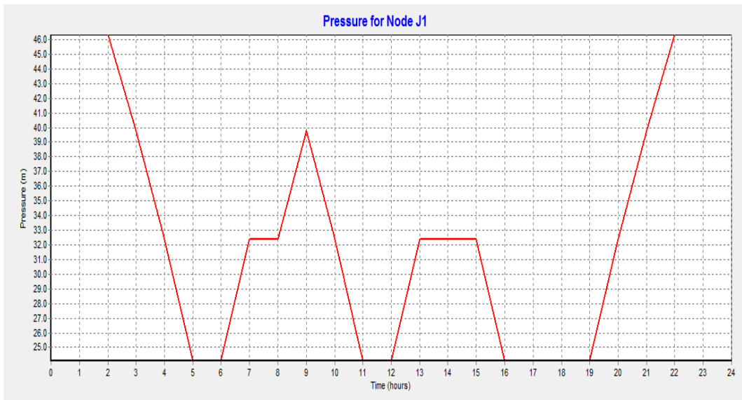
Gambar 6 Grafik Tekanan pada Junction J1
