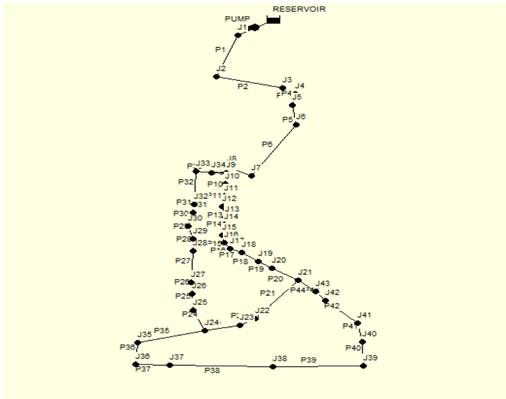
Gambar 3. Jaringan distribusi utama Sabak Auh
