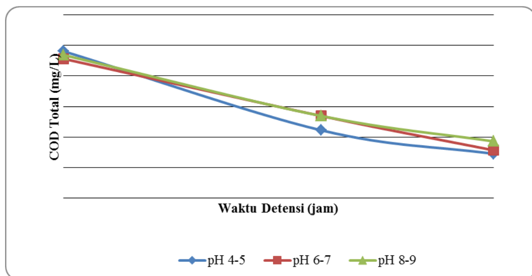
Gambar 2 Pengaruh pH terhadap COD
