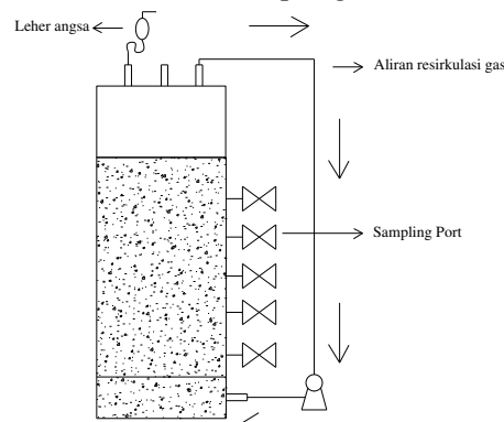
Gambar 1 Sketsa reaktor seeding aklimatisasi dan reaktor penelitian
