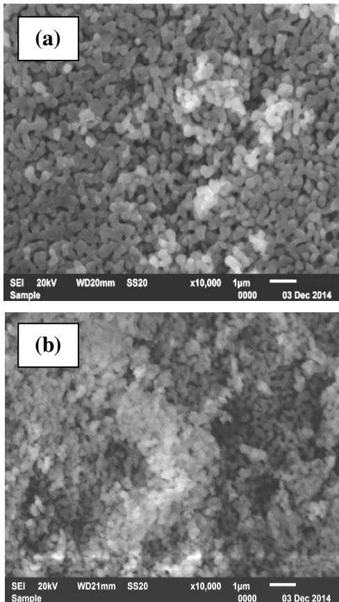
Gambar 3. Hasil SEM HAp sintesis dengan variasi rasio molar Ca/P (a) 0,67 dan (b) 2,67
