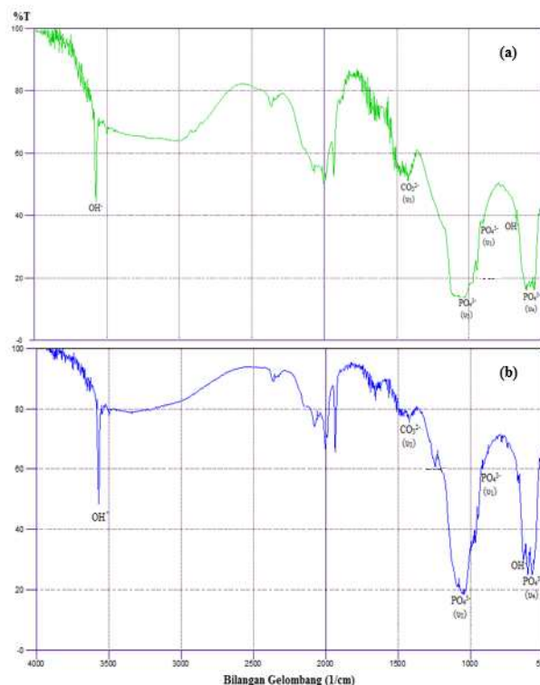
Gambar 2. Spektrum FTIR HAp sintesis dengan variasi rasio Ca/P (a) 0,67 dan (b) 2,67
