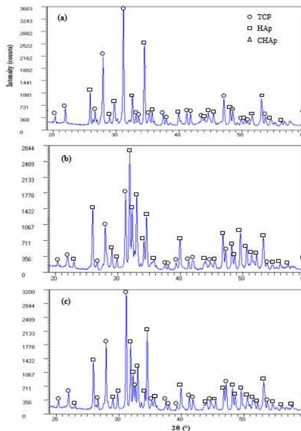
Gambar 1. Pola XRD HAP sintesis dengan rasio Ca/P (a) 0,67; (b) 1,67; dan (c) 2,67
