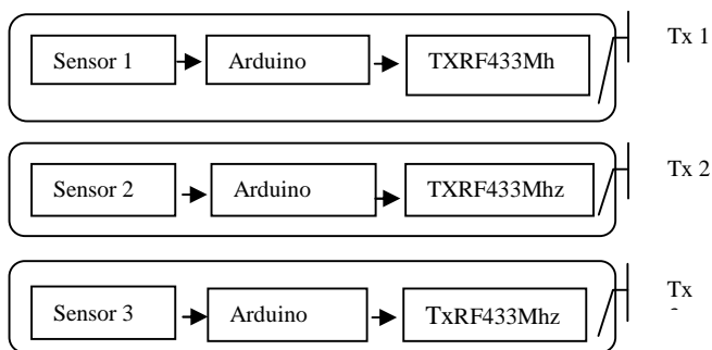
Gambar 5.1 Desain Rangkaian Transmitter
