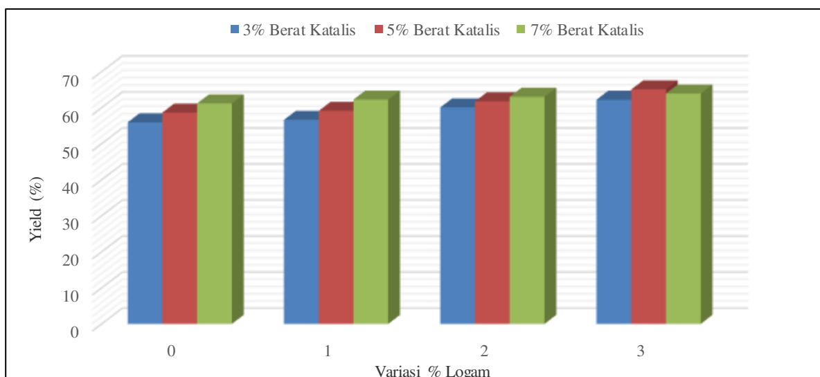
Gambar 3.1 Pengaruh Kadar Logam NiMo/NZA Terhadap Yield Bio-oil dengan Variasi Berat Katalis
