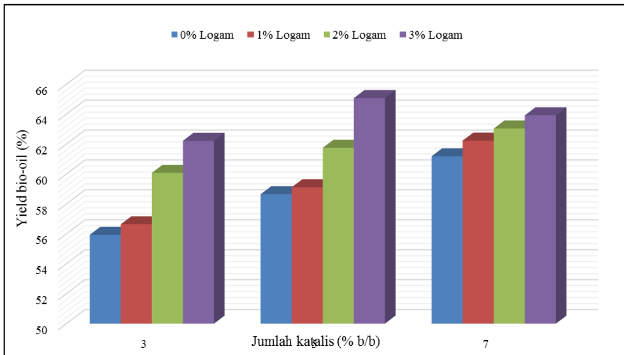
Gambar 3.3 Pengaruh Berat NiMo/NZA Terhadap Yield Bio-oil
