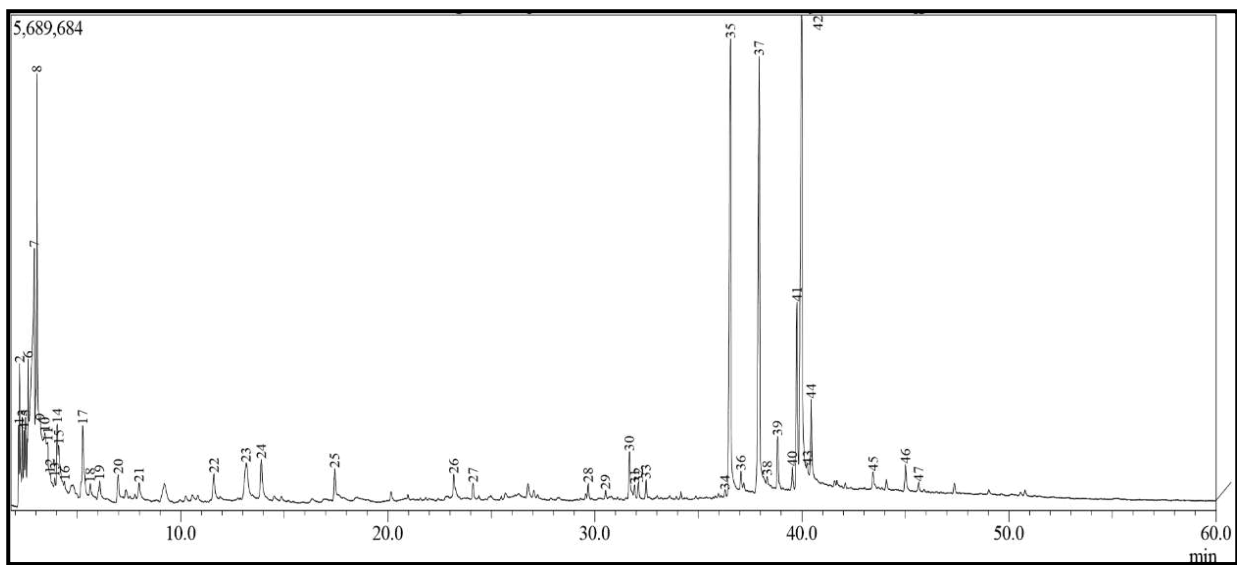
Gambar 3.4 Hasil Kromatogram Bio-oil Menggunakan Katalis NiMo/NZA 5% berat terhadap biomassa dengan Kadar Logam 3%
