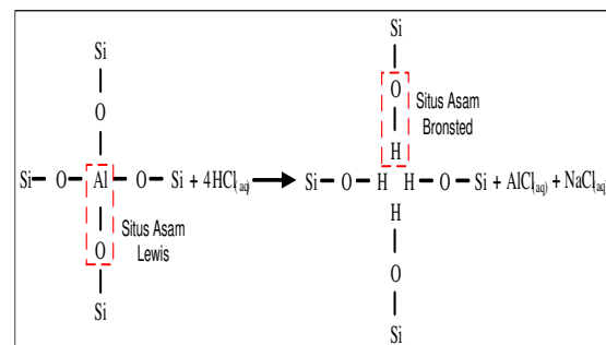
Gambar 3.2 Mekanisme Berkurangnya Situs Asam Lewis Dan Pembentukan Situs Asam Bronsted Pada Penambahan HCl
