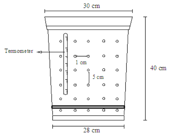
Gambar 2.1 Komposter
