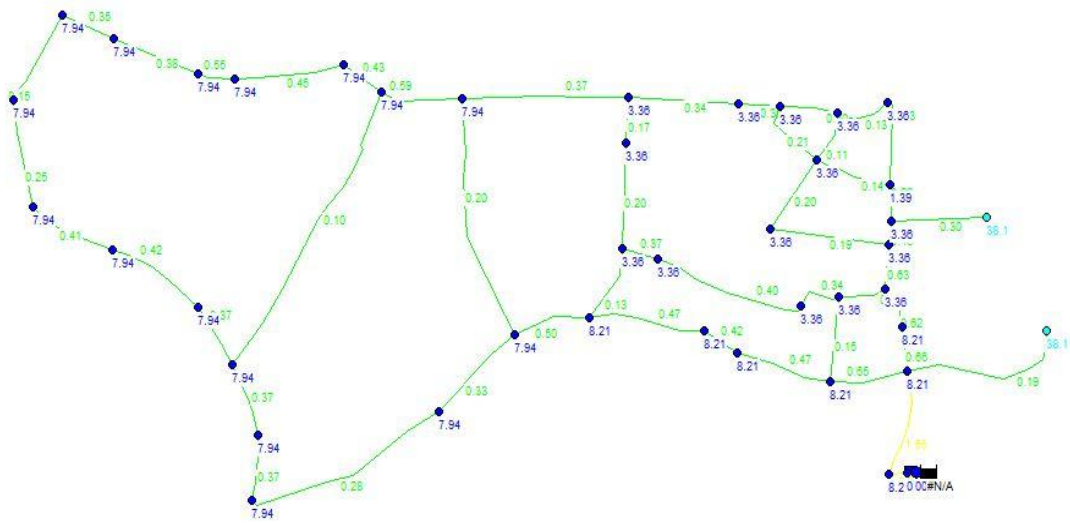
Gambar 4.3 Jalur Sistem Jaringan Distribusi
