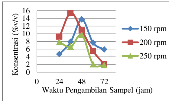
Gambar 3. Pengaruh Kecepatan Pengaduk Terhadap Konsentrasi Bioetanol Pada Kekentalan Nira 20%
