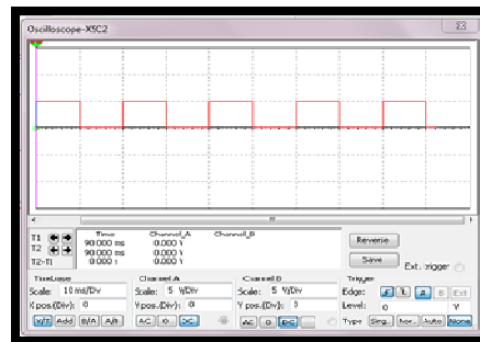
Gambar 10. Gelombang Keluaran Detektor Fasa Tanpa Beban Dan Tanpa Kapasitor
