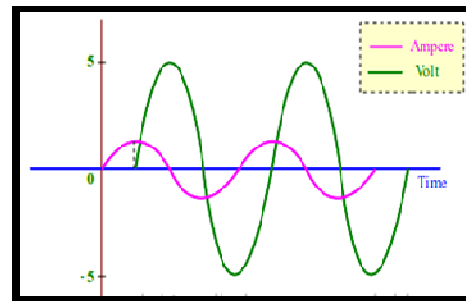
Gambar 6. Beban Kapasitif
