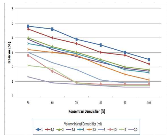
Gambar 1. Hubungan volume dan konsentrasi injeksi demulsifier terhadap BS&W
