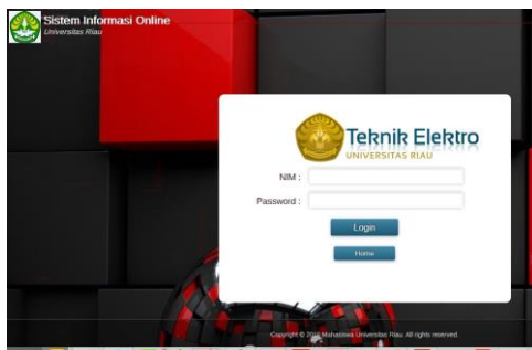
Gambar 3.1.3 Login Mahasiswa
