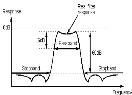
Gambar 3. Respon Filter dalam Praktiknya (Bowick, 1982)
