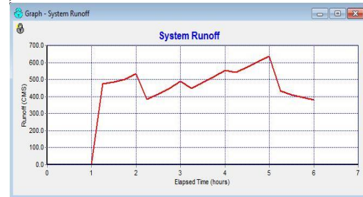
Gambar 3. Grafik Debit Banjir Kala Ulang 5 Tahun
