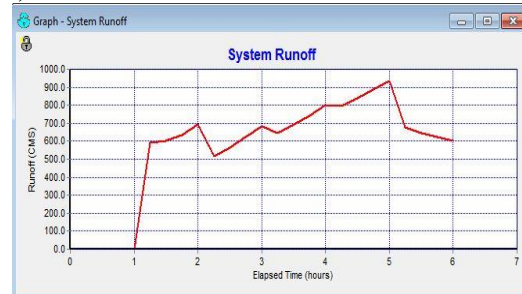
Gambar 4. Grafik Debit Banjir Kala Ulang 25 Tahun
