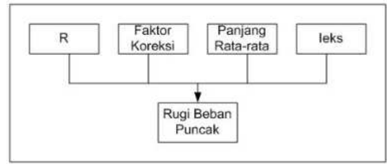
Gambar 15. Bagan Perhitungan Rugi Beban Puncak
