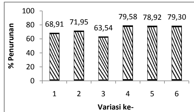
Gambar 3. Grafik persentase rata-rata penurunan nilai warna pada outlet biosand filter dual media
