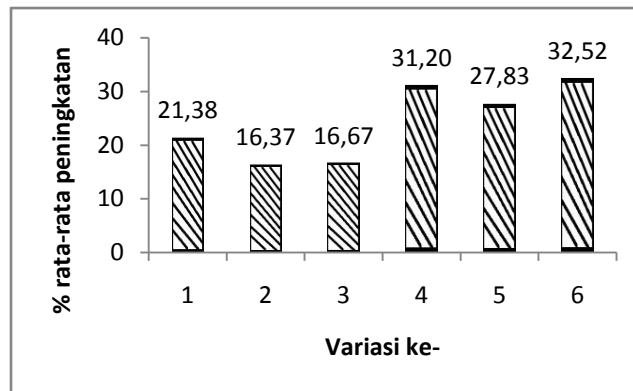
Gambar 1. Grafik persentase rata-rata peningkatan pH pada outlet biosand filter dual media.
