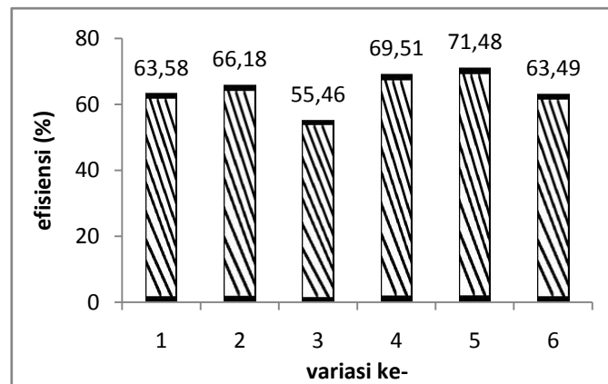
Gambar 4. Grafik persentase rata – rata penurunan nilai kandungan organik pada outlet biosand filter dual media
