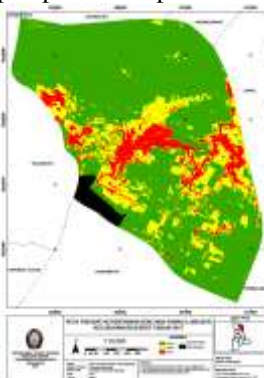
Gambar 9 Peta Tingkat Kerentanan Bencana Tanah Longsor
