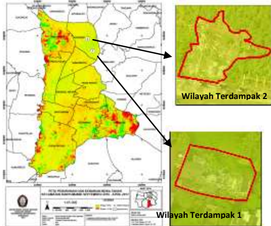
Gambar 15 Peta Penurunan dan Kenaikan Muka Tanah Terhadap Wilayah Terdampak Bencana Tanah Longsor
