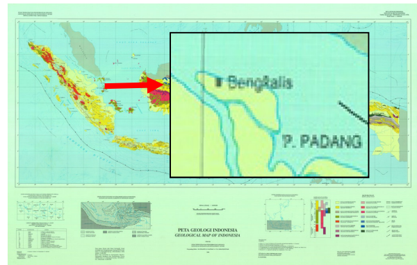
Gambar 7. Peta Geologi Indonesia (Sumber: Pusat Penelitian dan Pengembangan Geologi (1996))
