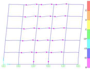
Gambar 12. Distribusi Sendi Plastis Langkah 2 pada Model 1
