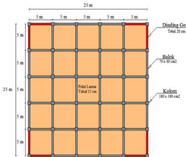
Gambar 6. Denah Lantai Pemodelan
