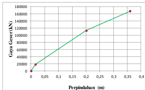
Gambar 9. Kurva Kapasitas Gedung Model 2
