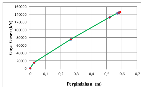
Gambar 10. Kurva Kapasitas Gedung Model 3
