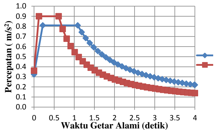
Gambar 7. Respon Spektrum Kota Banda Aceh
