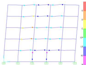
Gambar 13. Distribusi Sendi Plastis Langkah 4 pada Model 1
