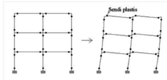
Gambar 5. Sendi Plastis yang Terjadi pada Balok dan Kolom
