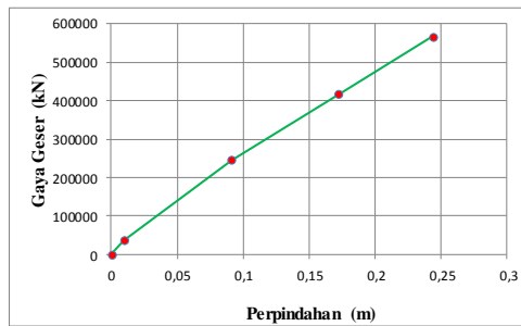
Gambar 8. Kurva Kapasitas Gedung Model 1
