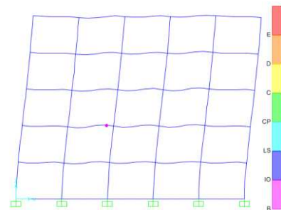
Gambar 11. Distribusi Sendi Plastis Langkah 1 pada Model 1
