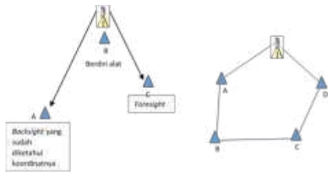
Gambar 5 Metode Traverse
