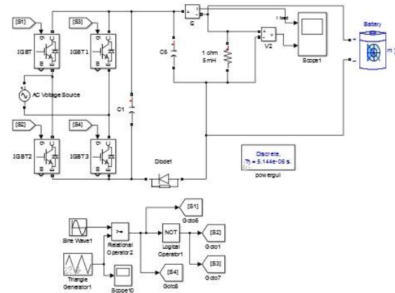
Gambar 4.3. Rangkaian Bidirectional Inverter Mode Penyearah
