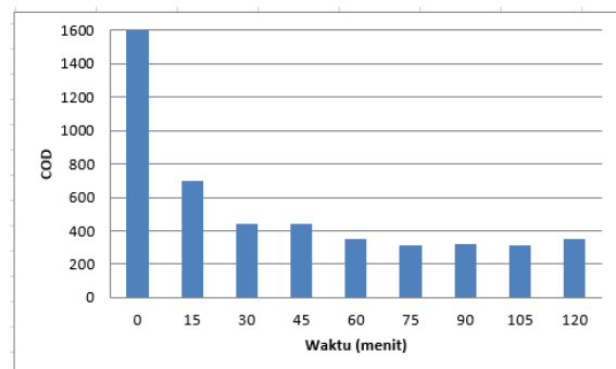
Gambar 1 Penurunan nilai COD terhadap waktu pada reaksi oksidasi
