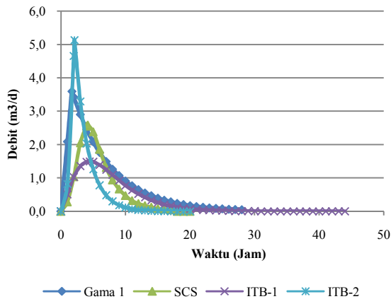
Gambar 8. Perbandingan Bentuk Hidrograf Empat Metode HSS Sub DAS Umban
