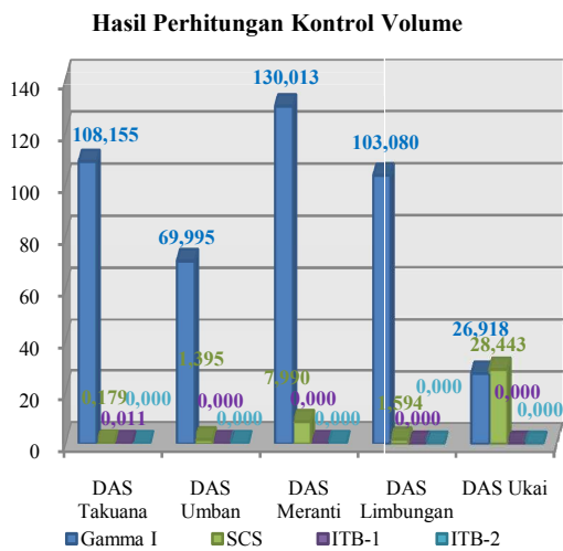
Gambar 9. Hasil Perhitungan Kontrol Volume
