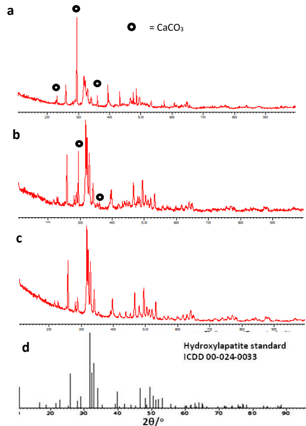
Gambar 3.4 Difraktogram HAp hasil sintesis pada suhu 140°C, waktu reaksi a) 12, b)16 dan c)20 jam, d)HAp standard (ICDD 00-024-0033)
