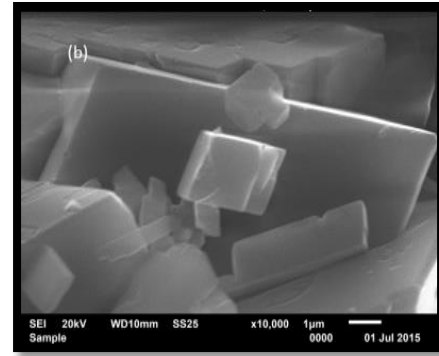
Gambar 3.2 Foto SEM PCC kulit kerang lokan (perbesaran 10000 x)
