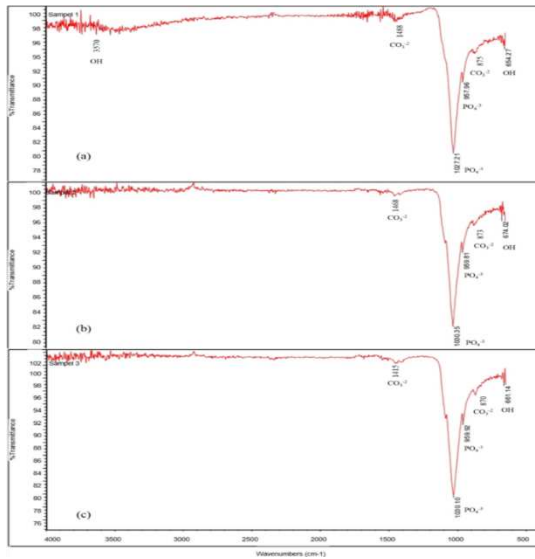
Gambar 3.3 Spektrum FTIR HAp hasil sintesis , waktu reaksi 12 jam dengan variasi suhu(a)140°C (b)160°C (c)180°C
