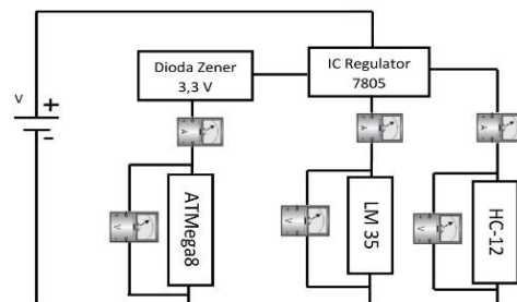
Gambar 6. Metode Pengukuran Tegangan Dan Arus Pada Prototipe di Lapangan
