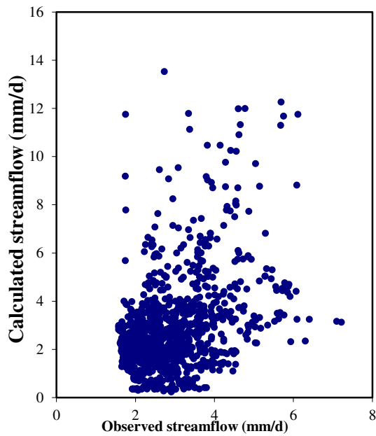
Gambar 11. Perbandingan debit kalkulasi dengan observasi kalibrasi skema 3
