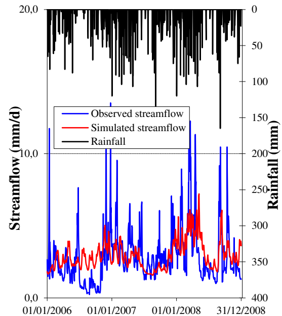
Gambar 9. Grafik hidograf kalibrasi skema 3
