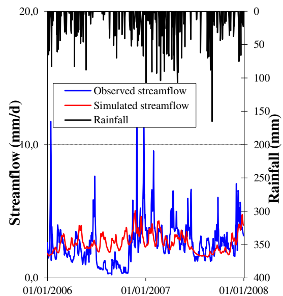
Gambar 10. Grafik hidograf verifikasi skema 2.a.
