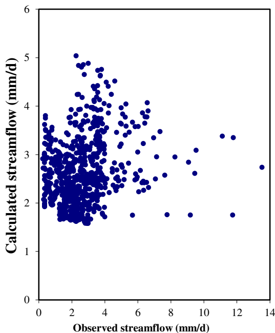
Gambar 12. Perbandingan debit kalkulasi dengan observasi kalibrasi skema 2.1
