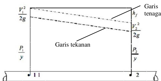
Gambar 3. Garis tenaga dan garis tekanan
