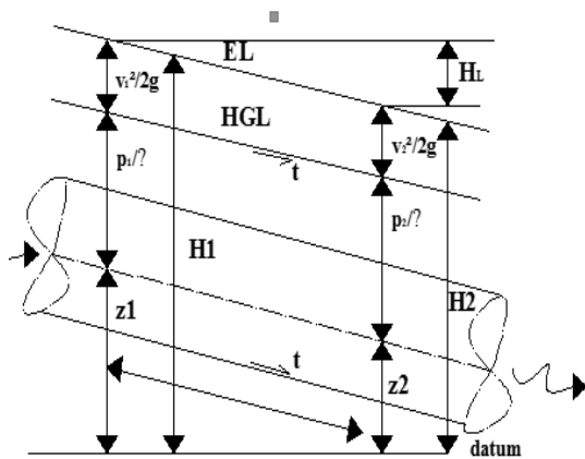
Gambar 1. Potongan memanjang pipa dengan jarak L relatif cukup jauh (sumber: Kodoatie, 2002)
