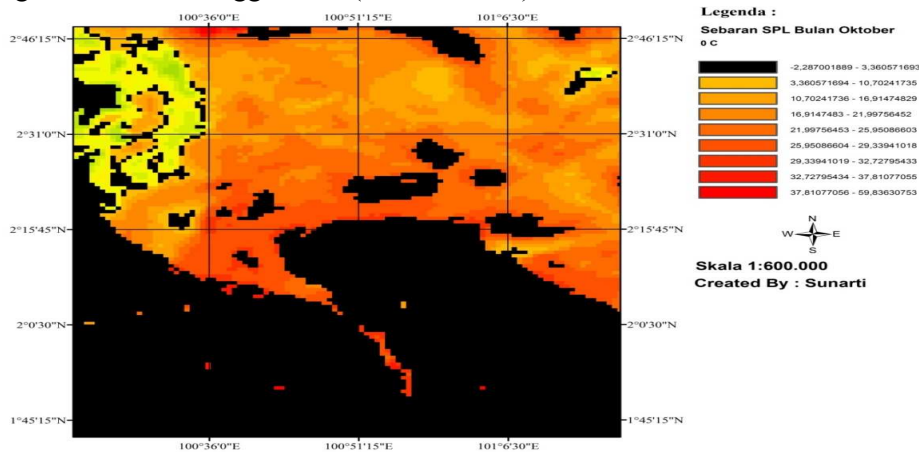
Gambar 7 : Sebaran SST di Perairan Rokan Hilir Bulan Oktober 2013 Sumber : Olahan data dari http://ladsweb.nasacom.nasa.gov
