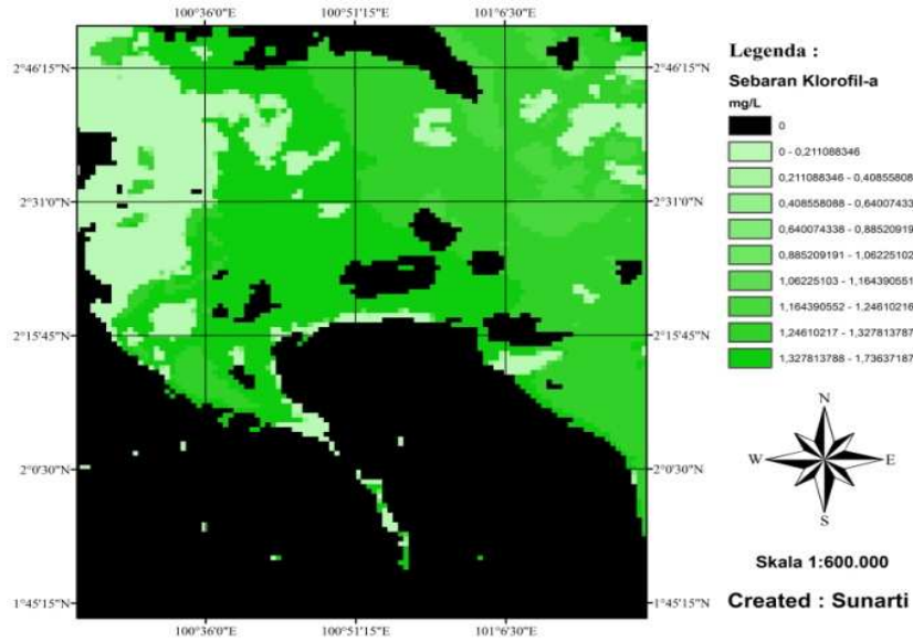
Gambar 4 : Sebaran Klorofil-a di Perairan Rokan Hilir Bulan Oktober 2013 Sumber : Olahan data dari http://ladsweb.nasacom.nasa.gov
