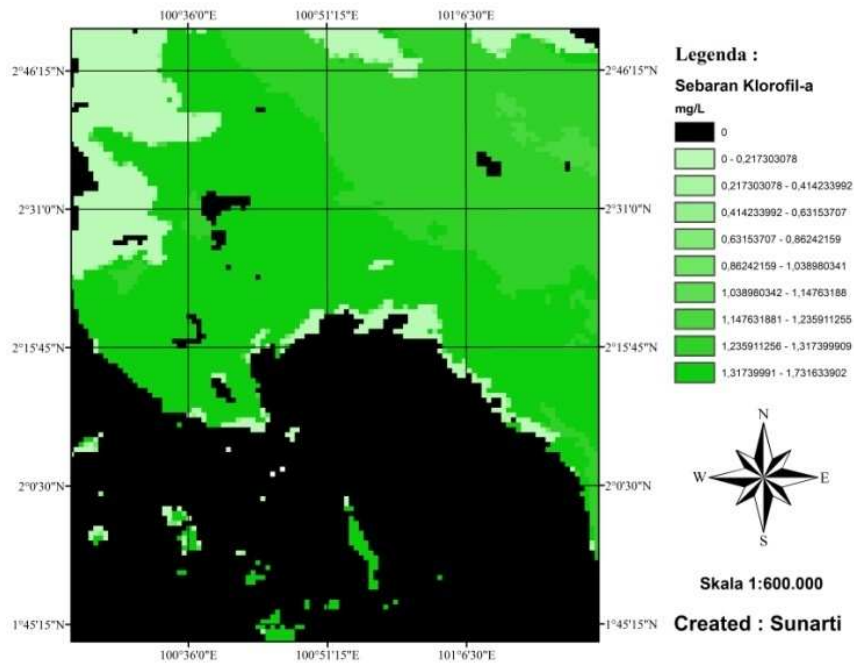
Gambar 5 : Sebaran Klorofil-a di Perairan Rokan Hilir Bulan November 2013 Sumber : Olahan data dari http://ladsweb.nasacom.nasa.gov
