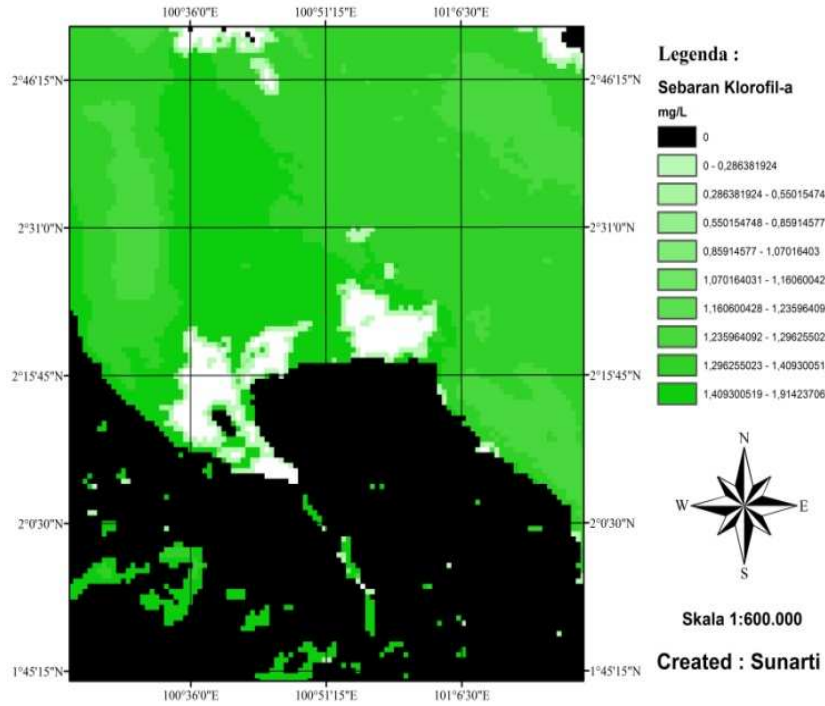
Gambar 6: Sebaran Klorofil-a di Perairan Rokan Hilir Bulan Desember 2013 Sumber : Olahan data dari http://ladsweb.nasacom.nasa.gov
