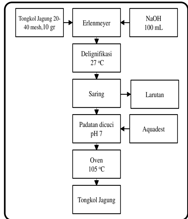
Gambar 2.1 Diagram Alir Pembuatan Enzim
