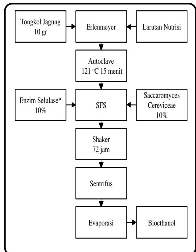
Gambar 2.2 Diagram Alir Pembuatan Bioetanol
