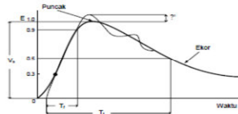
Gambar 3. Bentuk Tegangan Impuls Petir
