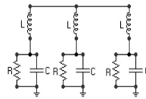
Gambar 13. Model Rangkaian dengan Tiga Elektroda Pentanahan
