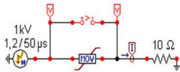
Gambar 10. Rangkaian Sederhana Arrester MOV
