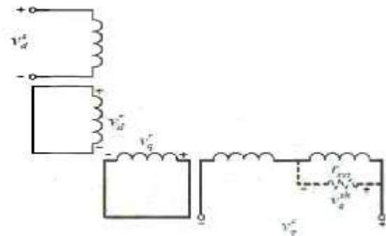
Gambar 3.9 model motor yang belitannya terhubung singkat pada stator
