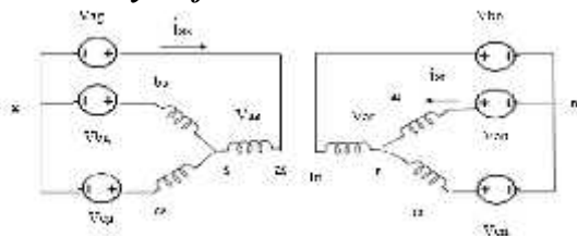
Gambar 3.2 Hubungan stator dan rotor
