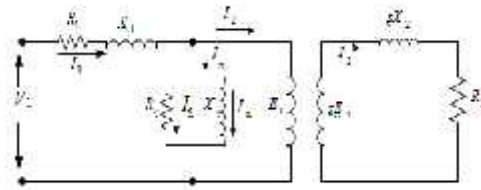
Gambar 2.2 Rangkaian Ekvivalen Motor Induksi
