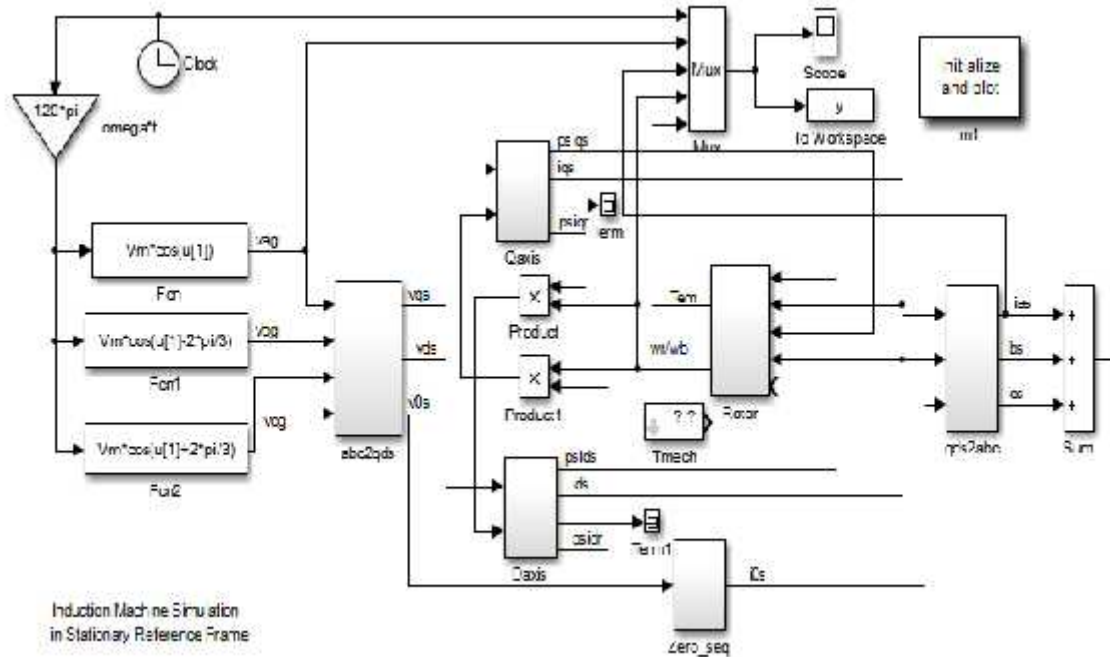
Gambar 4.3 Model motor induksi tiga fasa dalam Kerangka Referensi Stationer
