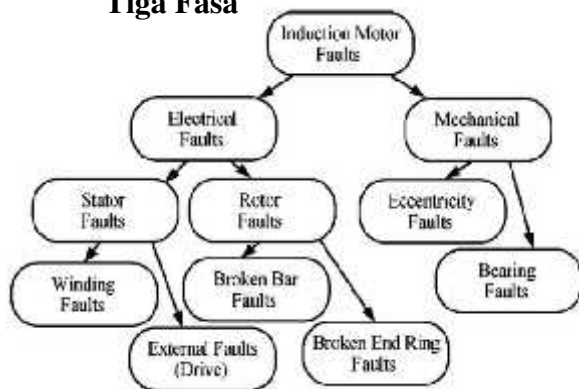
Gambar 2.3. Klasifikasi gangguan motor induksi tiga fasa
